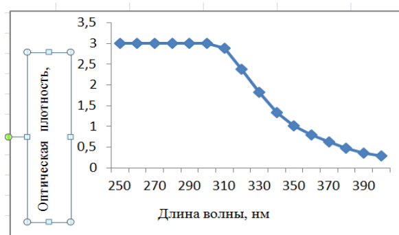
Рис. 3. УФ-спектр исходного фильтрата отбелки целлюлозы (раствор сравнения — вода)
